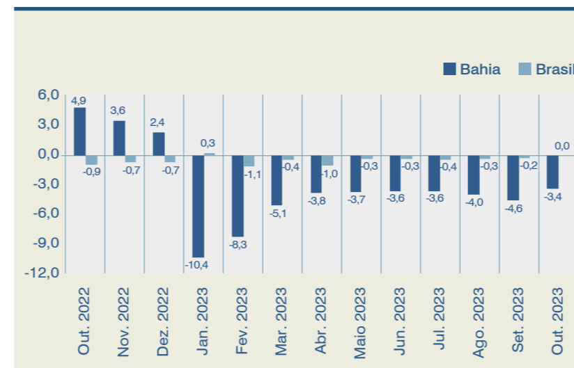
Gráfico 3 – Produção física industrial(1) – Bahia e Brasil – Out. 2022-out. 2023
