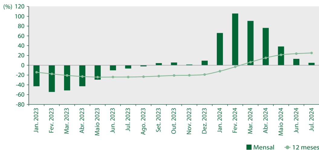
Gráfico 3 Produção de petróleo – Bahia – Jan. 2023-jul. 2024
