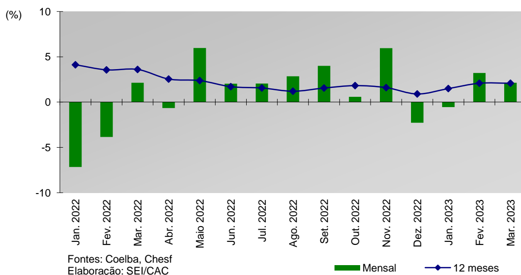
Gráfico 5 – Consumo de energia elétrica – Bahia – Jan. 2022 - Mar. 2023
